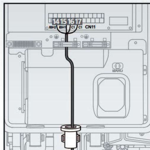
IBH (Interní záložní ohřivač) 9 kW
