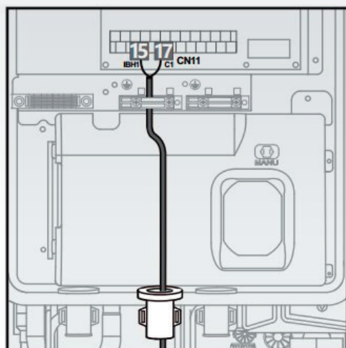
IBH (Interní záložní ohřivač) 3 kW
