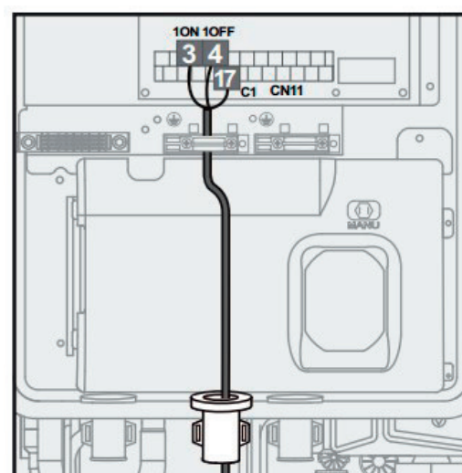
SV1 (3-cestný ventil pro TUV)
