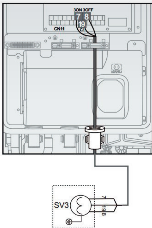
SV3 (3-cestný mixovací ventil pro druhou zónu)
