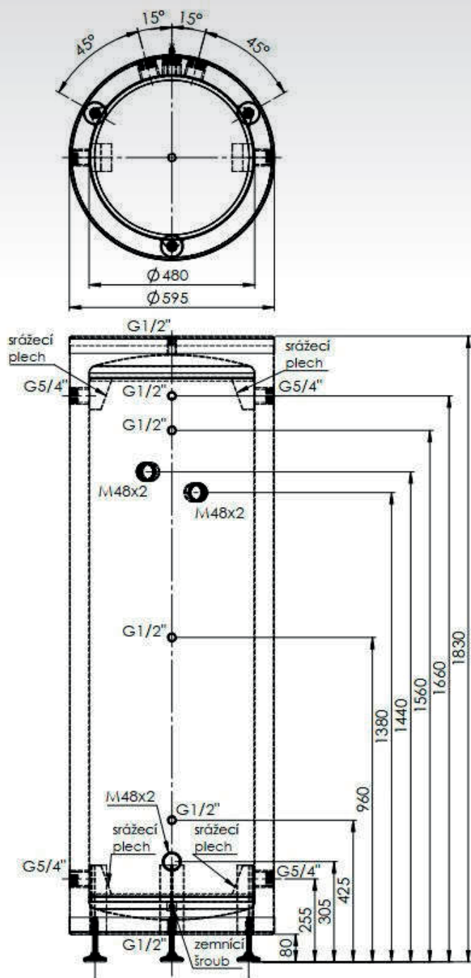
AKU ST 300 S
