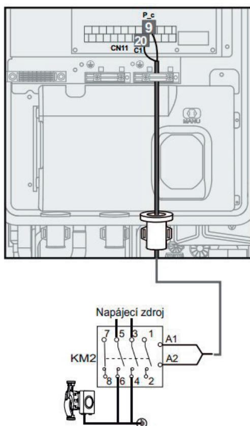
Oběhové čerpadlo 2 zóny
