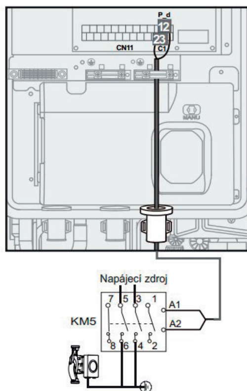
Oběhové čerpadlo pro cirkulaci TUV
